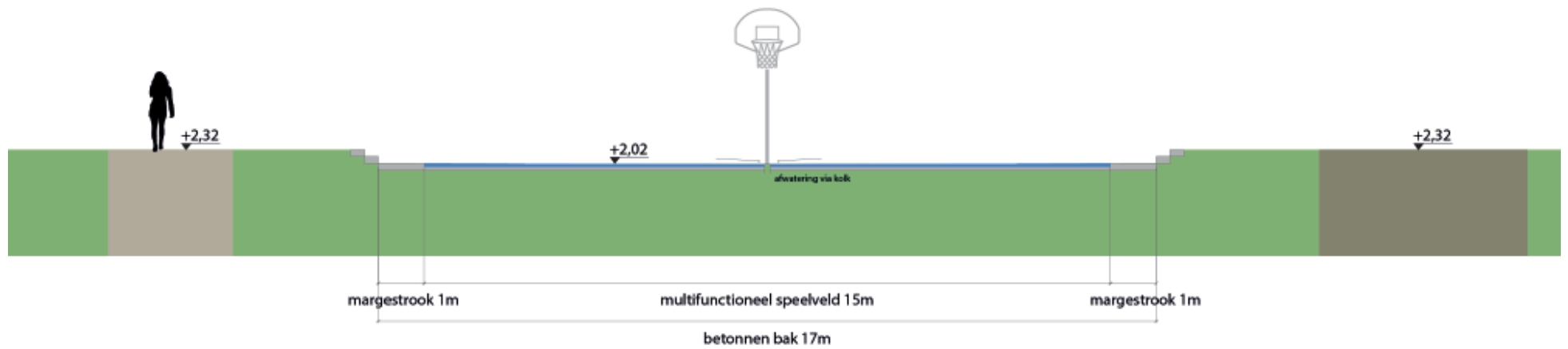
Doorsnede multifunctioneel sportveldje wanneer het verhard wordt.
