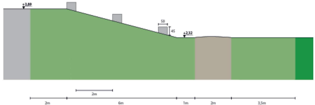
Doorsnede tribune, afmetingen elementen in millimeters.
