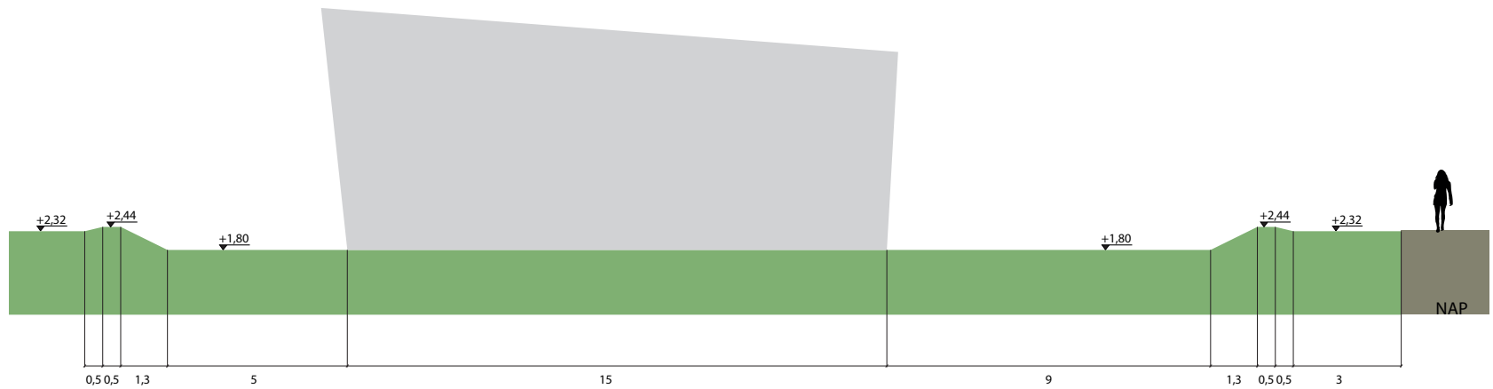
Principeprofiel van de booster in dwarsrichting
